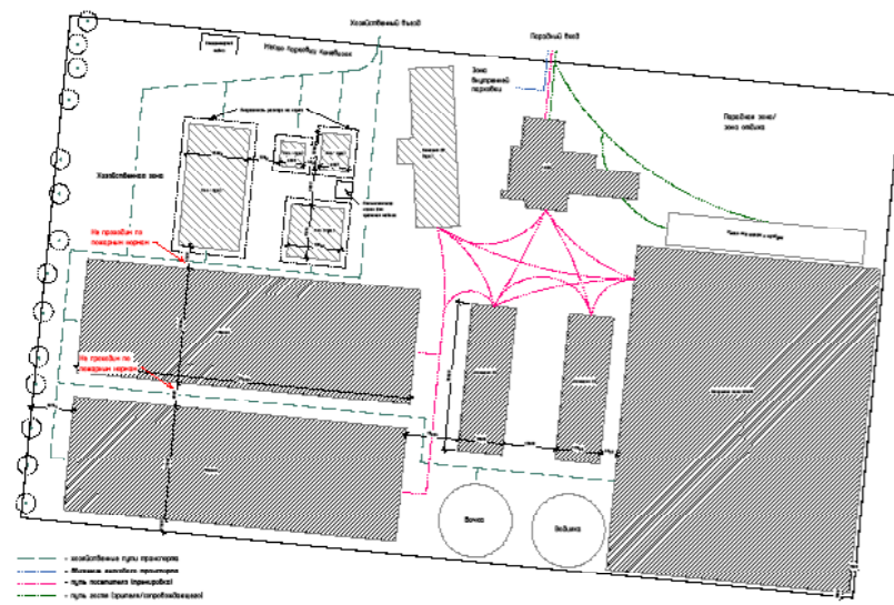
Функциональная схема
